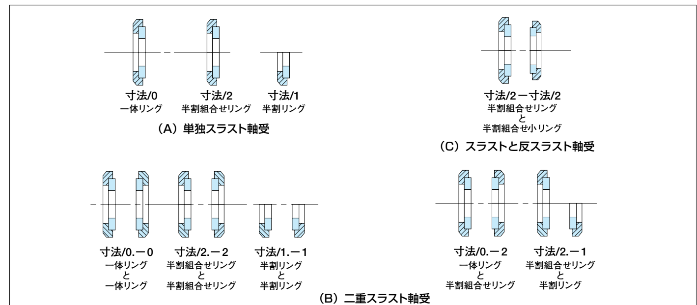
図6 - 軸受の一般的な組合せとその識別記号
